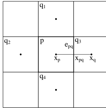
Obr. 2: Detail siete spolu s označením. V strede sa nachádza pixel p , susedné pixle sú označené ako q_i , kde q_i = 1, 2, 3, 4 , hrany medzi pixlami označíme ako e_{pq} , x_p a x_q sú reprezentatívne body.
