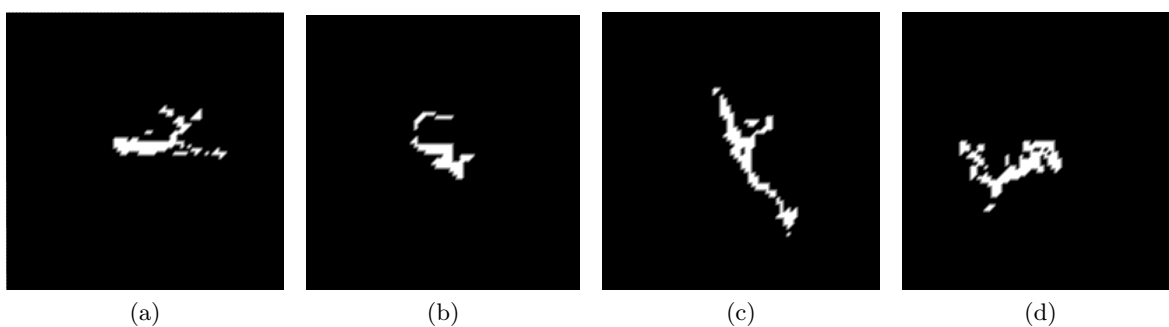
Obr. 25: Bernsenova metóda.
